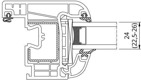
Listwa 50924
