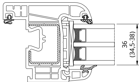
Listwa 50936
