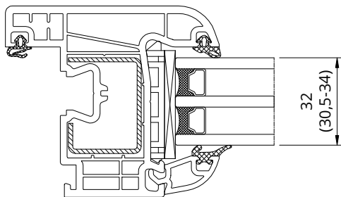
Listwa 50932
