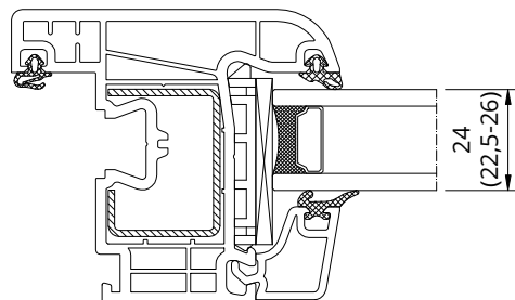
Listwa 50924A
