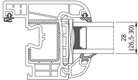
Listwa 50928
