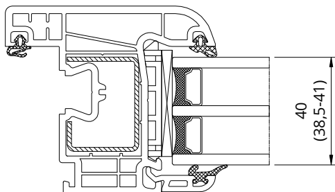
Listwa 50940
